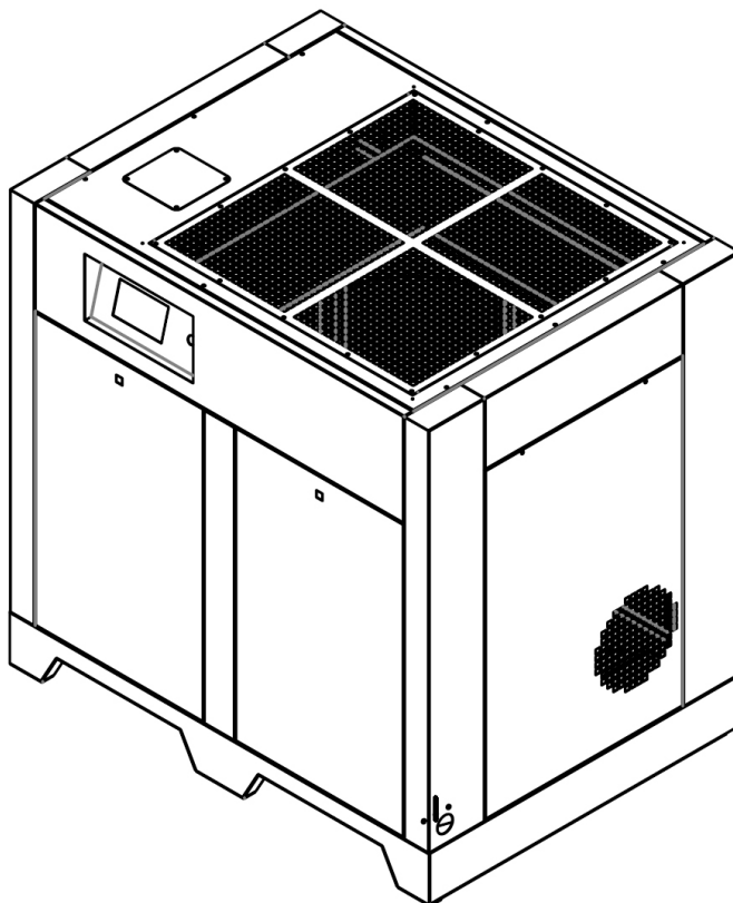
Рис. 3.1 Вид снаружи винтового компрессора серии XB
